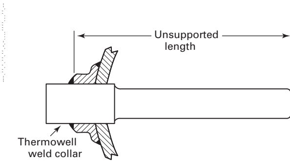
(b) Socket Weld Thermowell
