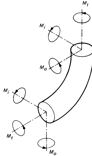
Fig. 519.4.5-1 Bends
