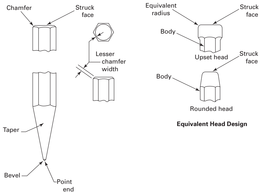
Fig. 1 Nomenclature for Type II Punches
