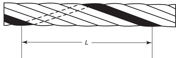
Fig. 1.3.3.2.1-1 Strand Lay Length
