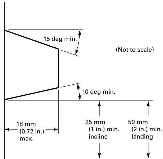
Fig. 6.1.3.3.10 Dimensions
