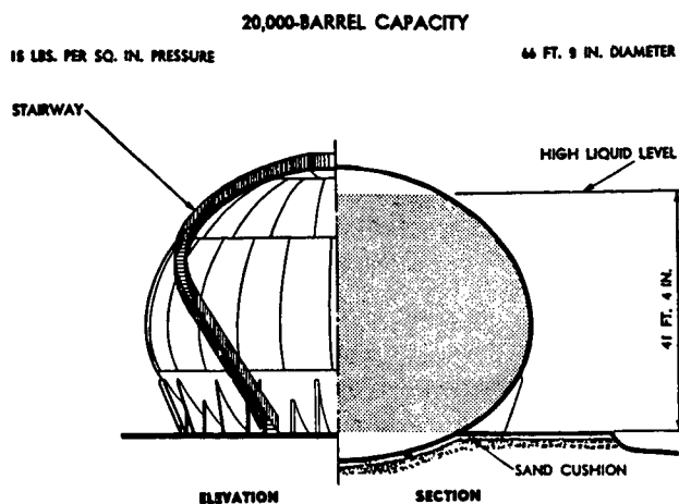
FIG. 1—Spheroid.
