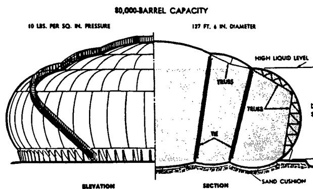
FIG. 2—Noded Spheroid.
