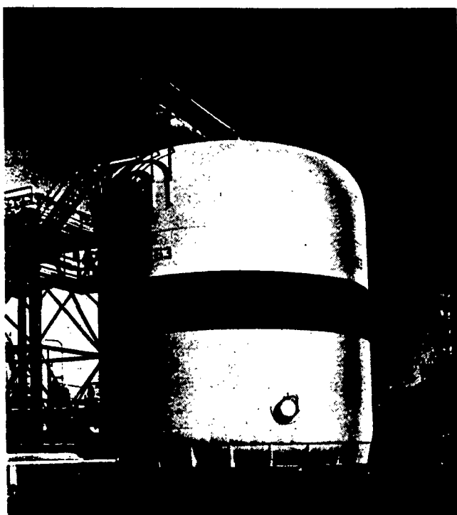
FIG. 3—Ellipsoid.
