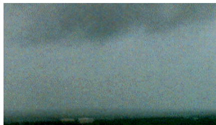
Nimbostratus
