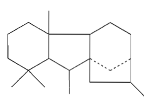
Fig. 6.58. Gibberellane
