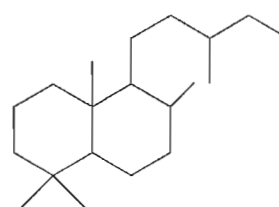
Fig. 6.53. Labdane
