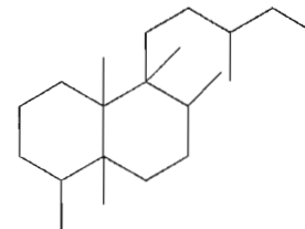
Fig. 6.54. Clerodane
