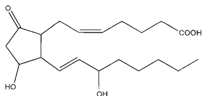
Fig. 5.4. Prostaglandin E 2
