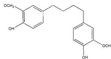
Fig. 7.67. Dihydroguaiaretic acid
