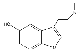
Fig. 8.25. Bufotenine
