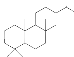
Fig. 6.56. Abiatane
