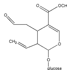
Fig. 8.24. Secologanin
