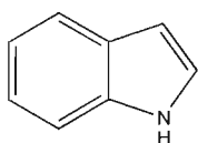
Fig. 8.22. Indole
