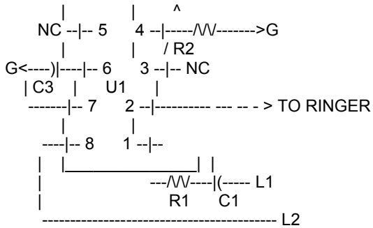
a. Main ringer TTL circuit
