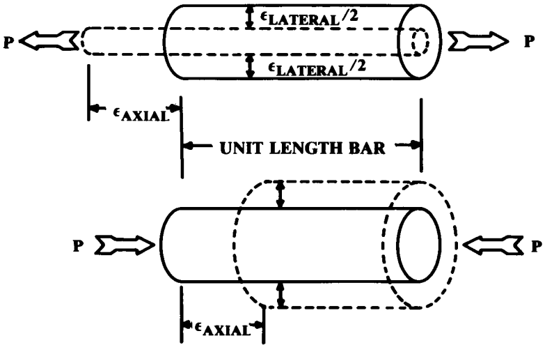
Fig. 14.19 Poisson's ratio.
