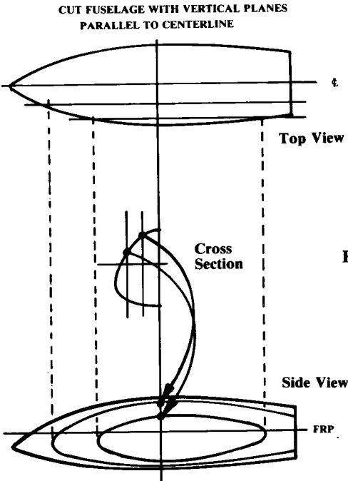
Fig. 7.21 Buttock-plane cut.
