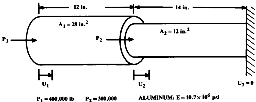
Fig. 14.49 FEM example.
