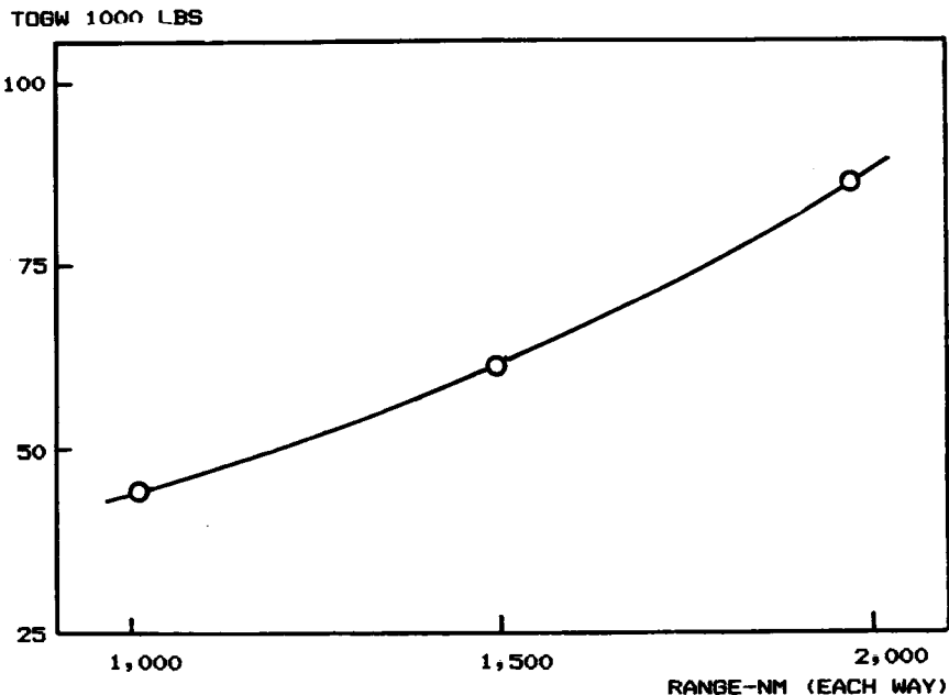
Fig. 3.11 Range trade.
