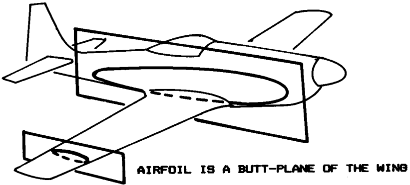
Fig. 7.21 Buttock-plane cut.
