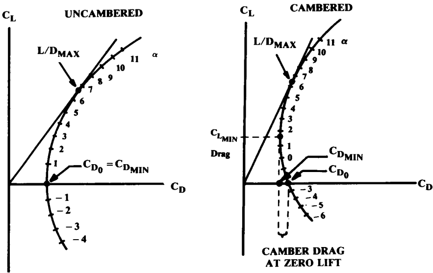
Fig. 12.3 Drag polar.
