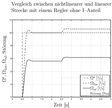
Abb. 12.32: \Omega_{lin} und \Omega_{nl} bei Regelung ohne I-Anteil und \kappa = 15 Vergleich zwischen nichtlinearer und linearer Strecke mit einem Regler ohne I-Anteil
