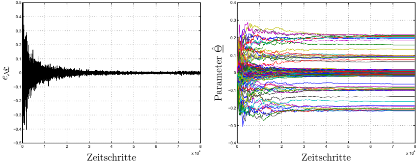
Abb. 9.12: Identifikation mit Beobachter — Fehlerverlauf (links) und Konvergenz der Parameter (rechts)
