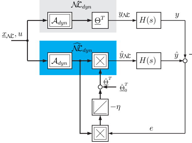
Abb. 9.7: Lerngesetz nach Fehlermodell 3 zur Adaption von \widehat{N}_{\mathcal{L}_{dyn}}
