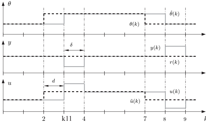
Abb. 15.13: Parameter, Regelgröße und Stellgröße bei Regelung mit multiplen Modellen
