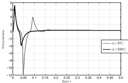
(c) Stellgröße
