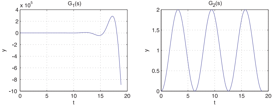
Abb. 16.1: Sinusantwort der unregelten Strecken (16.17) und (16.18).
