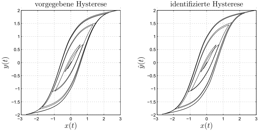
Abb. 5.43: Vorgegebene (links) und identifizierte (rechts) Hysteresis
