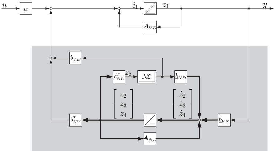
Abb. 16.22: Signalflussplan des Gesamtsystems, bestehend aus nichtlinearem Zweimassensystem und DT_1 -Filter, in Byrnes-Isidori-Normalform.
