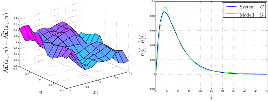
Abb. 9.17: Identifikationsfehler der statischen Nichtlinearität (links) und identifizierte Impulsantwort (rechts)
