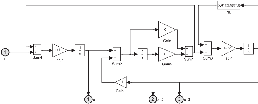
Abb. 5.9: Simulink-Modell des nichtlinearen Zweimassensystems
