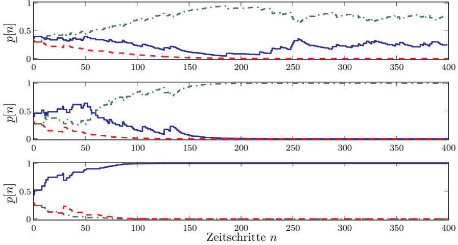
Abb. 15.7: Lernprozess unter dem L_{R-I} -Algorithmus mit Lernschrittweiten a = 0.05/0.1/0.15 (von oben nach unten). p_1[n] (—), p_2[n] (---), p_3[n] (---)
