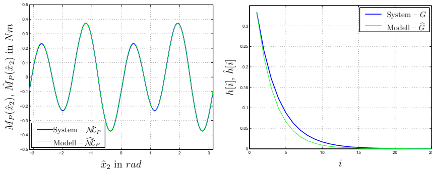
Abb. 9.26: Identifikationsergebnis der periodischen Nichtlinearität (links) und der identifizierten Impulsantwort (rechts)
