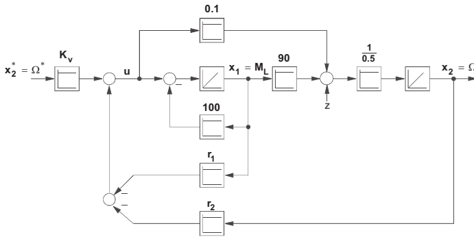
Abb. 12.28: Signalflußplan des linearen Vergleichregelkreises
