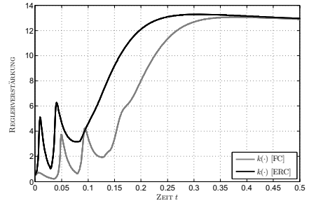
(d) Reglerverstärkung
