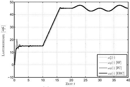
(a) Lastdrehzahl
