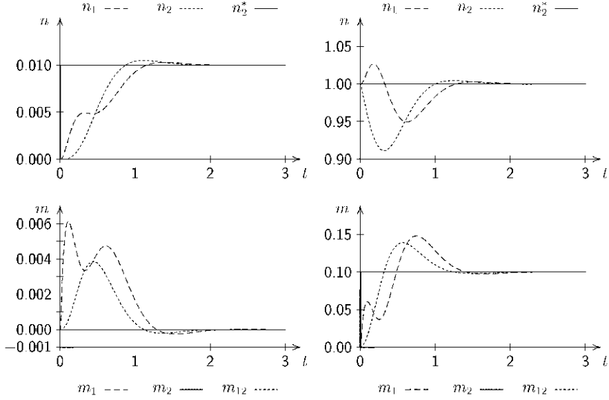
Abb. 2.20: Zustandsregelung mit I -Anteil bei \omega_{0(N)} = 6.2832 \text{ s}^{-1} (weiche Kopplung)
