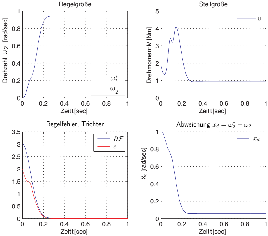
Abb. 16.24: Regelung des Zweimassensystems mit Berücksichtigung des Verdrehwinkels mittels Zustandsauskopplung c = \begin{pmatrix} 1 & 50 & 1 \end{pmatrix} ; k_{\Delta\varphi} = 50 , konstant.
