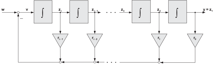
Abb. 12.14: Regelgesetz mit Integratorkette
