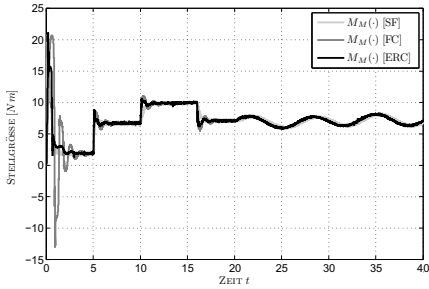
(c) Stellgröße
