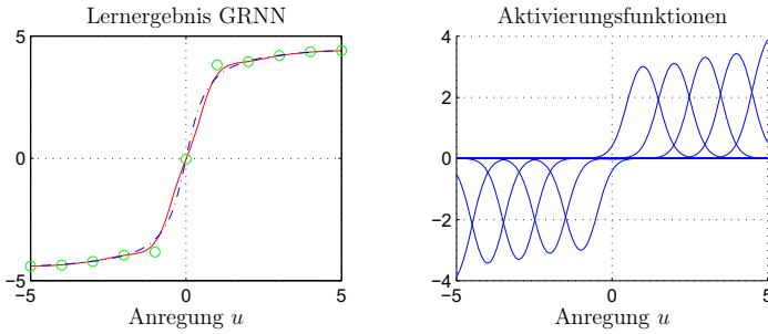
Abb. 3.11: Gelernte Kennlinie (—) mit den einzelnen Gewichten ( \circ ) und wahre Kennlinie (---) (links) und Aktivierungsfunktionen (rechts) für \sigma_{norm} = 0.5
