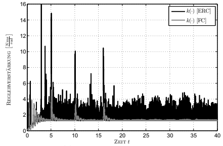
(f) Reglerverstärkung
