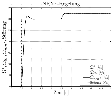
Abb. 12.42: Drehzahlverläufe bei Regelung nach NRNF
