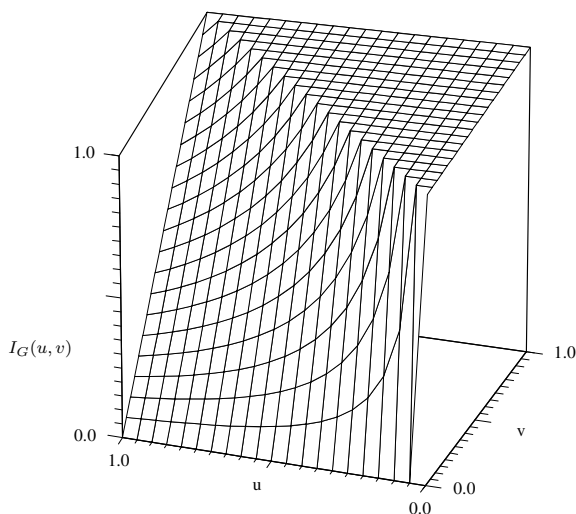
Abb. 18.52: Gaines-Implikation
