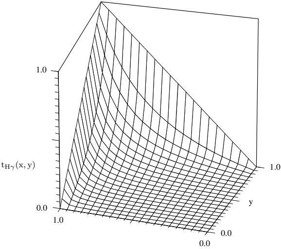
Abb. 18.29: Hamacher-Durchschnittsoperator, \gamma = 50
