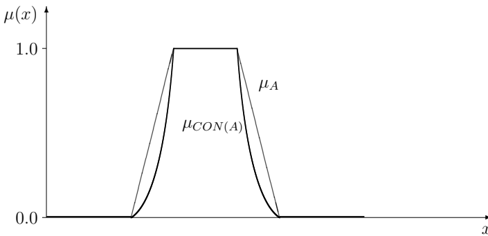
Abb. 18.9: Konzentrationsoperator
