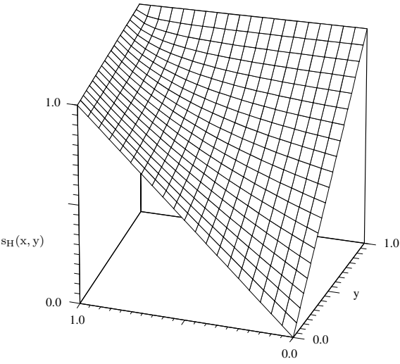
Abb. 18.21: Hamacher-Summe
