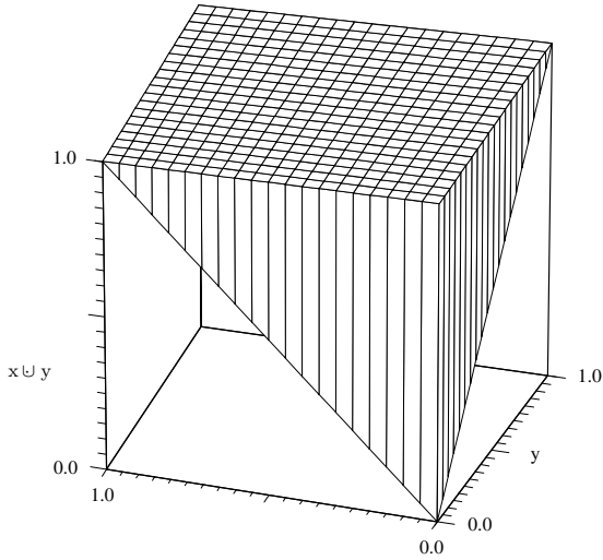
Abb. 18.25: Drastische Summe
