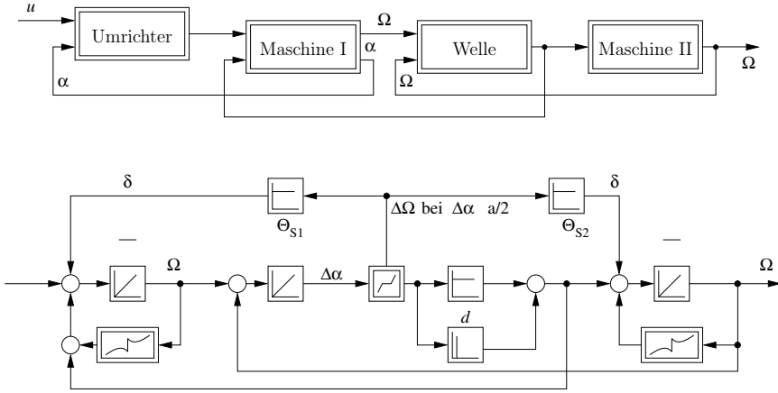
Abb. 6.18: Struktur des Systems (oben) und Signalflußplan des Zweimassensystems unter Vernachlässigung des Umrichters (unten)
