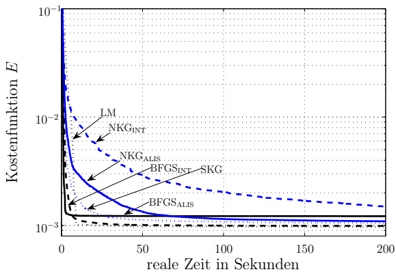
Abb. 10.32: Konvergenzverläufe bei der Identifikation der verrauschten Messdaten von Abbildung 10.31 mit einem 1-5-5-1-MLP.
