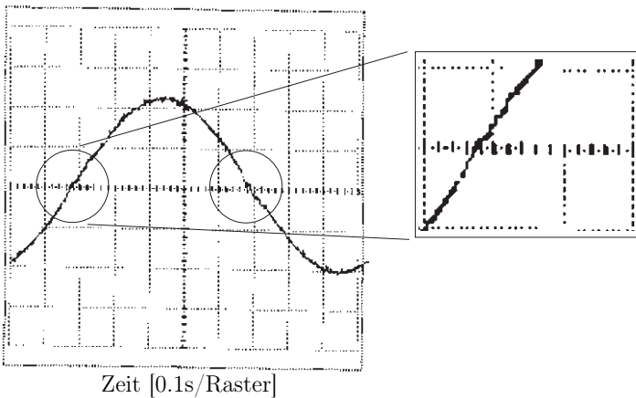
Abb. 5.35: Berechnete Schlittengeschwindigkeit mit Reibungskompensation
