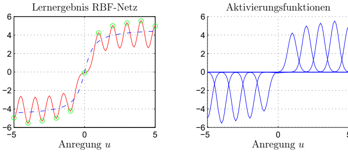
Abb. 3.9: Gelernte Kennlinie (—) mit den einzelnen Gewichten (○) und wahre Kennlinie (—) (links) und Aktivierungsfunktionen (rechts) für p = 11 Stützpunkte und \sigma_{norm} = 0.3
