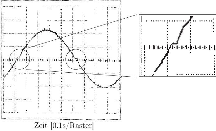
Abb. 5.34: Berechnete Schlittengeschwindigkeit ohne Reibungskompensation
