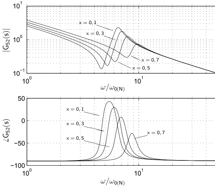
Abb. 2.7: Bode-Diagramm zu G_{S2}(s) : Variation des Trägheitsmomentenverhältnis x
