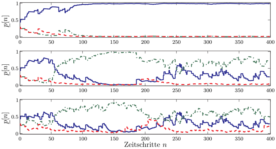
Abb. 15.9: Lernprozess unter dem L_{R-\varepsilon P} -Algorithmus mit a = 0.15 und \varepsilon = 0.01/0.05/0.15 (von oben nach unten). p_1[n] (—), p_2[n] (---), p_3[n] (- -)
