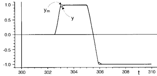
Abb. 12.58: Simulationsergebnisse. y(t) und y_m(t) stimmen nicht mehr exakt überein. Der Eingangsräum verlässt den gelernten Bereich.
