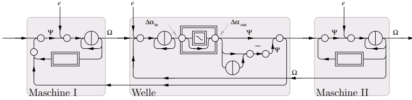
Abb. 6.19: Strukturiertes rekurrentes Netz für das losebehaftete Zweimassensystem
