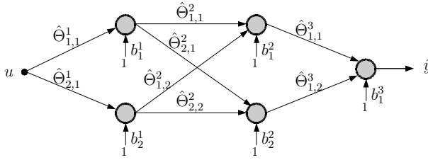
Abb. 4.8: Beispiel-MLP zur Identifikation der \arctan -Kennlinie von Abbildung 4.7
