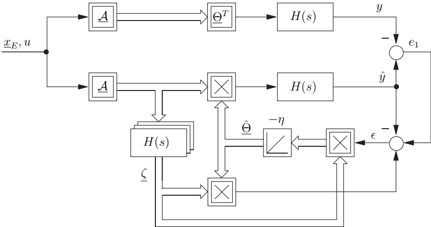
Abb. 5.19: Fehlermodell 4
