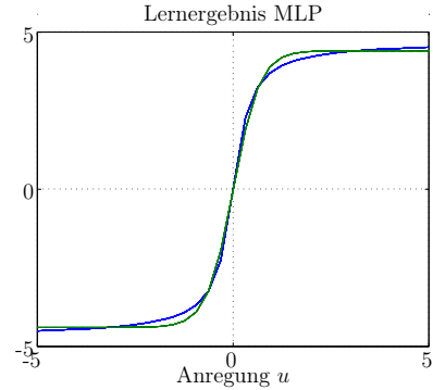
Abb. 3.57: Gelernte Kennlinie (---) und wahre Kennlinie (-)
