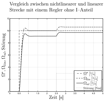
Abb. 12.31: \Omega_{lin} und \Omega_{nl} bei Regelung ohne I-Anteil und \kappa = 3 Vergleich zwischen nichtlinearer und linearer Strecke mit einem Regler ohne I-Anteil
