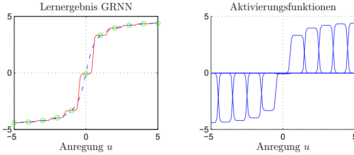
Abb. 3.13: Gelernte Kennlinie (-) mit den einzelnen Gewichten ( \circ ) und wahre Kennlinie (.-) (links) und Aktivierungsfunktionen (rechts) für \sigma_{norm} = 0.2
