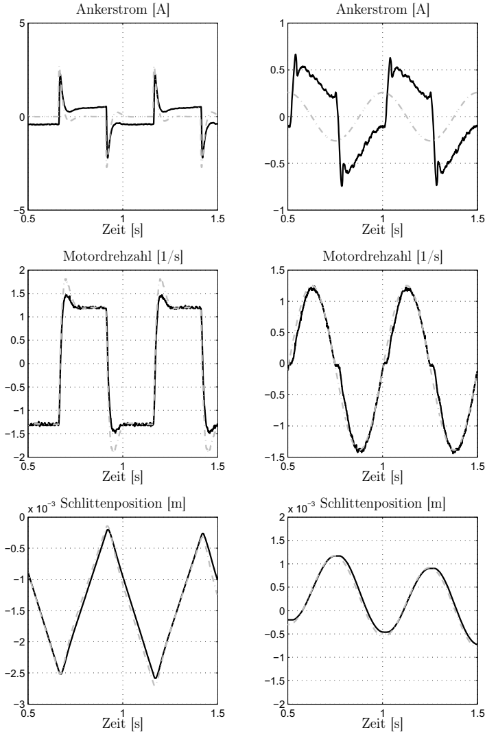
Abb. 2.21: Vergleich von simuliertem linearem Modell und gemessenen Daten (schwarz: Gemessene Daten; grau: Simulations Daten)
