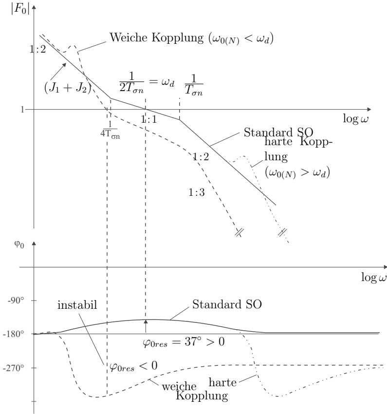
Abb. 2.5: Frequenzgänge des offenen \varphi_2 -Regelkreises
