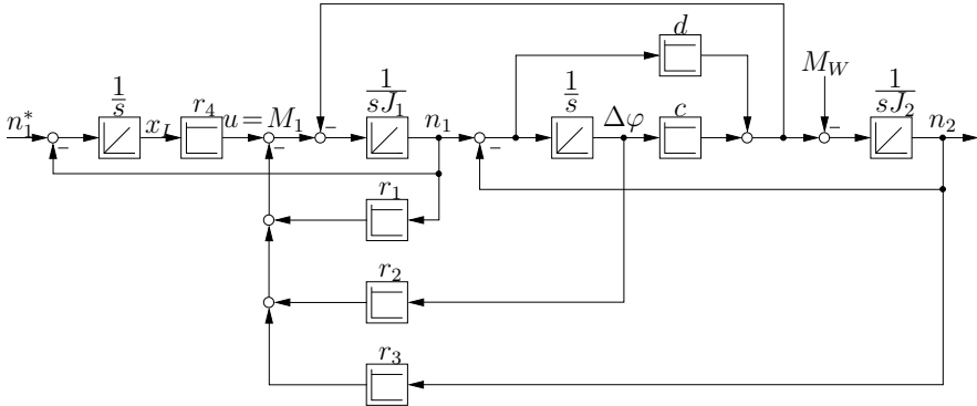
Abb. 2.17: Signalflußplan der Zustandsregelung mit I -Anteil
