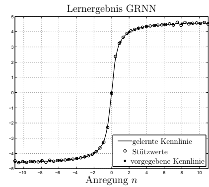
Abb. 12.50: identifizierte Nichtlinearität \mathcal{NL}(x_E)
