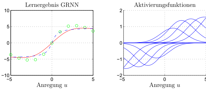
Abb. 3.12: Gelernte Kennlinie (—) mit den einzelnen Gewichten ( \circ ) und wahre Kennlinie (---) (links) und Aktivierungsfunktionen (rechts) für \sigma_{norm} = 1.5
