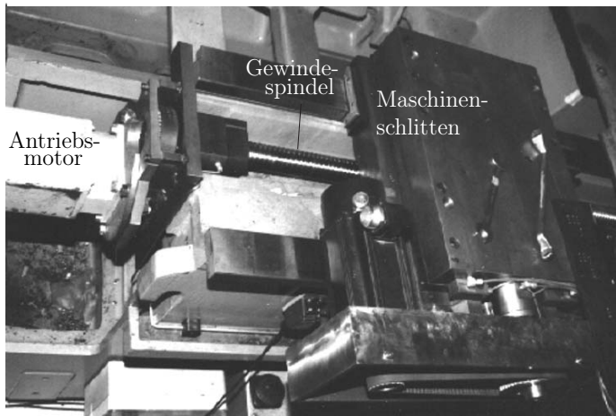
Abb. 5.20: Vorschubantrieb
