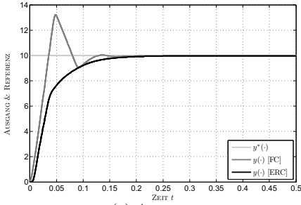
(a) Ausgang
