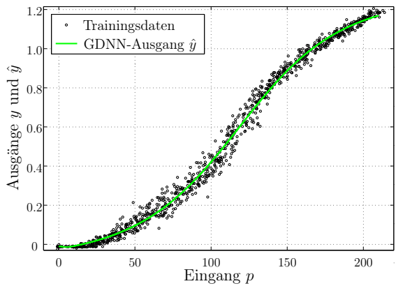
Abb. 10.33: Validierung der identifizierten Kennlinie mit den gegebenen Messdaten nach einer LM-Identifikation von 3 Sekunden.
