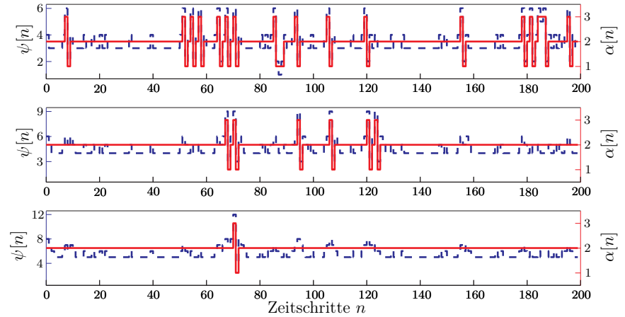
Abb. 15.11: Lernprozess dreier L_{3m,3} -Automaten mit Gedächtnistiefe m = 2/3/4 . Zustand \psi[n] (- -) und Aktion \alpha[n] (—)
