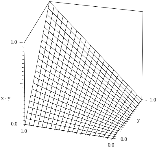
Abb. 18.16: Algebraisches Produkt
