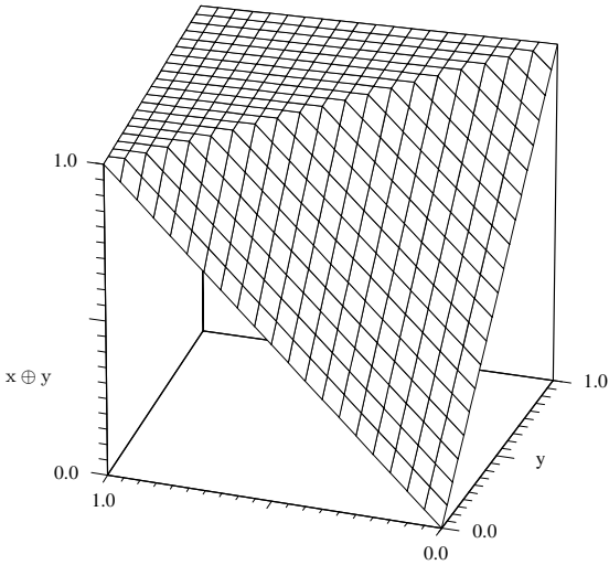
Abb. 18.24: Beschränkte Summe
