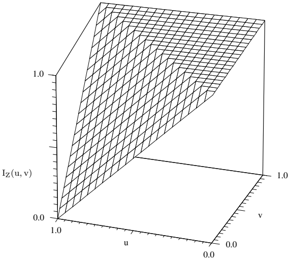
Abb. 18.48: Arithmetische Implikation
