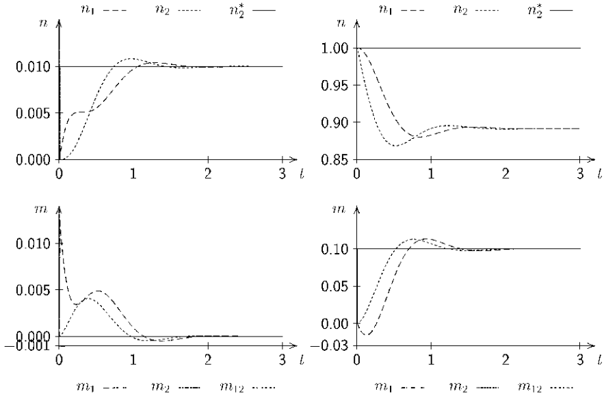
Abb. 2.16: Zustandsregelung ohne I -Anteil bei \omega_{0(N)} = 6.2832 \text{ s}^{-1} (weiche Kopplung)
