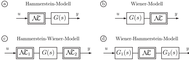
Abb. 8.2: Blockorientierte nichtlineare Modelle
