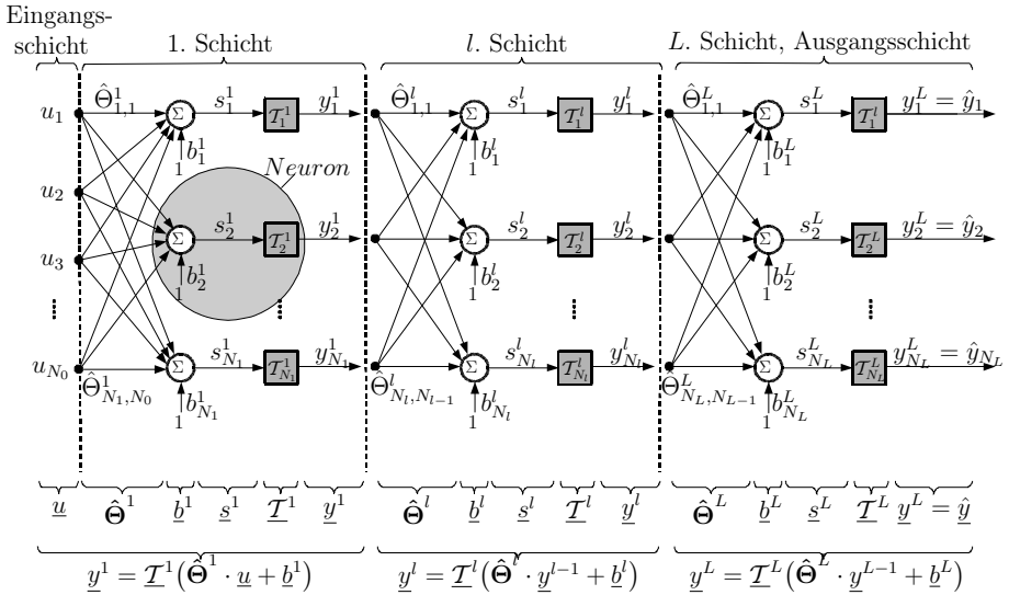
Abb. 3.48: Ein allgemeines feedforward Netzwerk mit L trainierbaren Schichten
