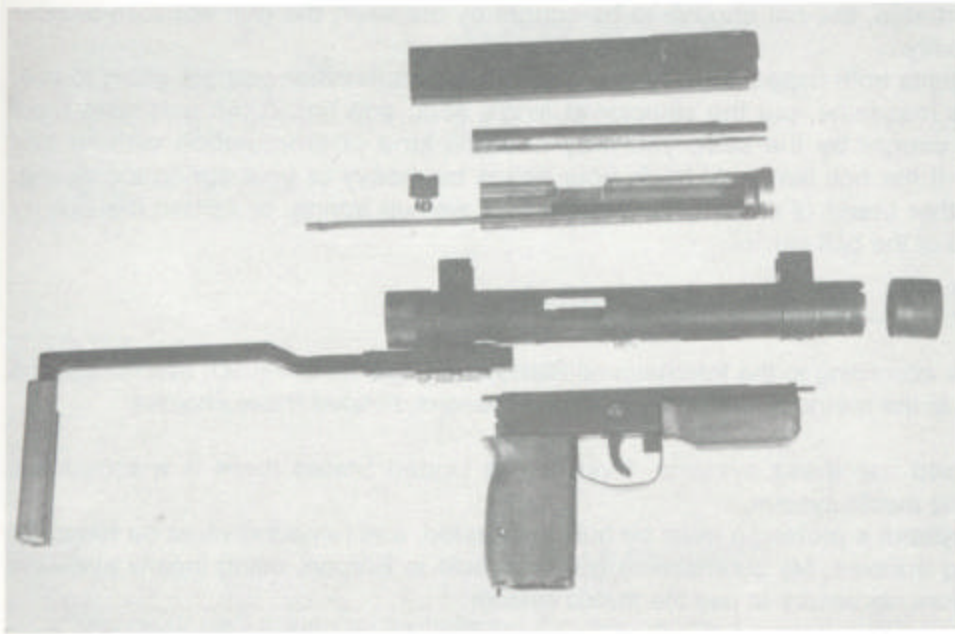
Field-stripped Métral.
