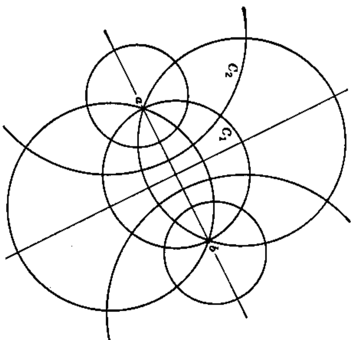
FIG. 3-3. Steiner circles.
