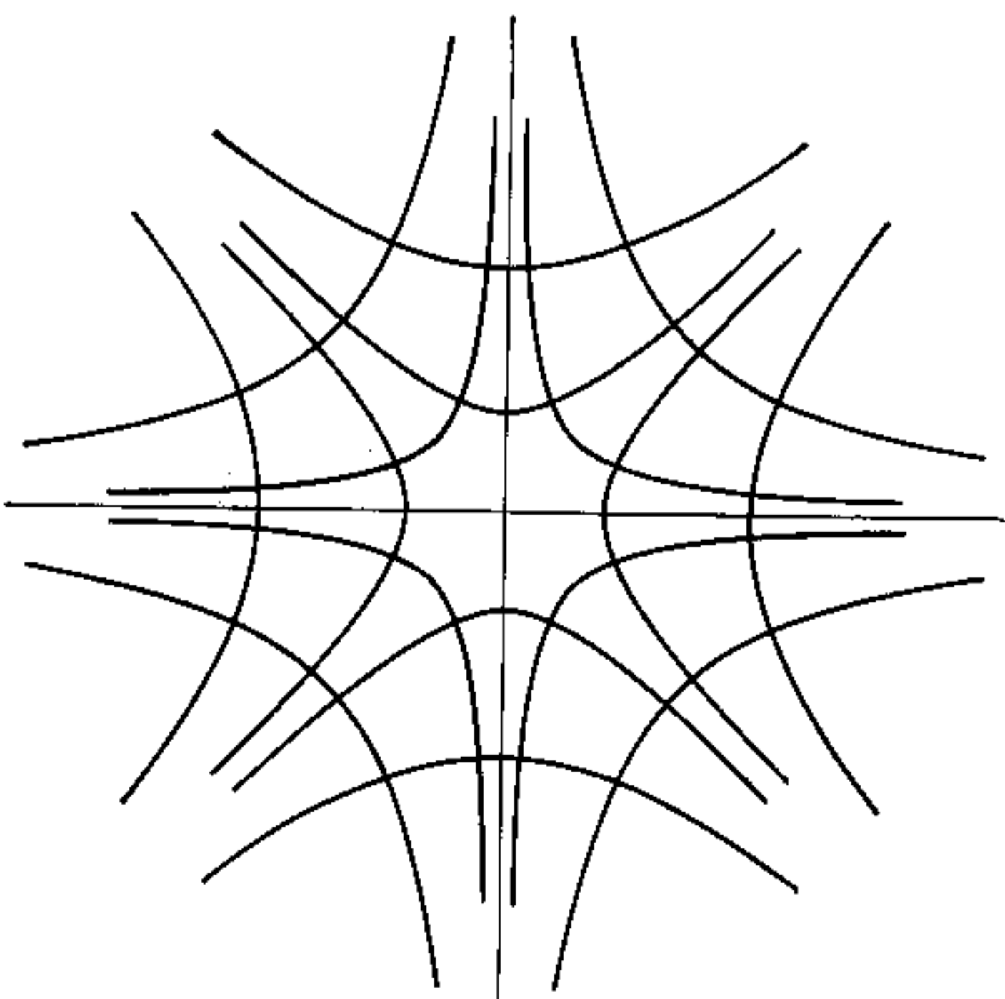
FIG. 3-5. z -plane.
