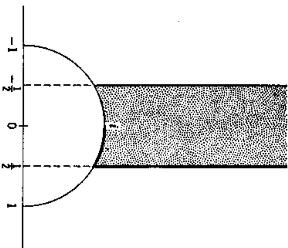
FIG. 7-2. z -plane.
