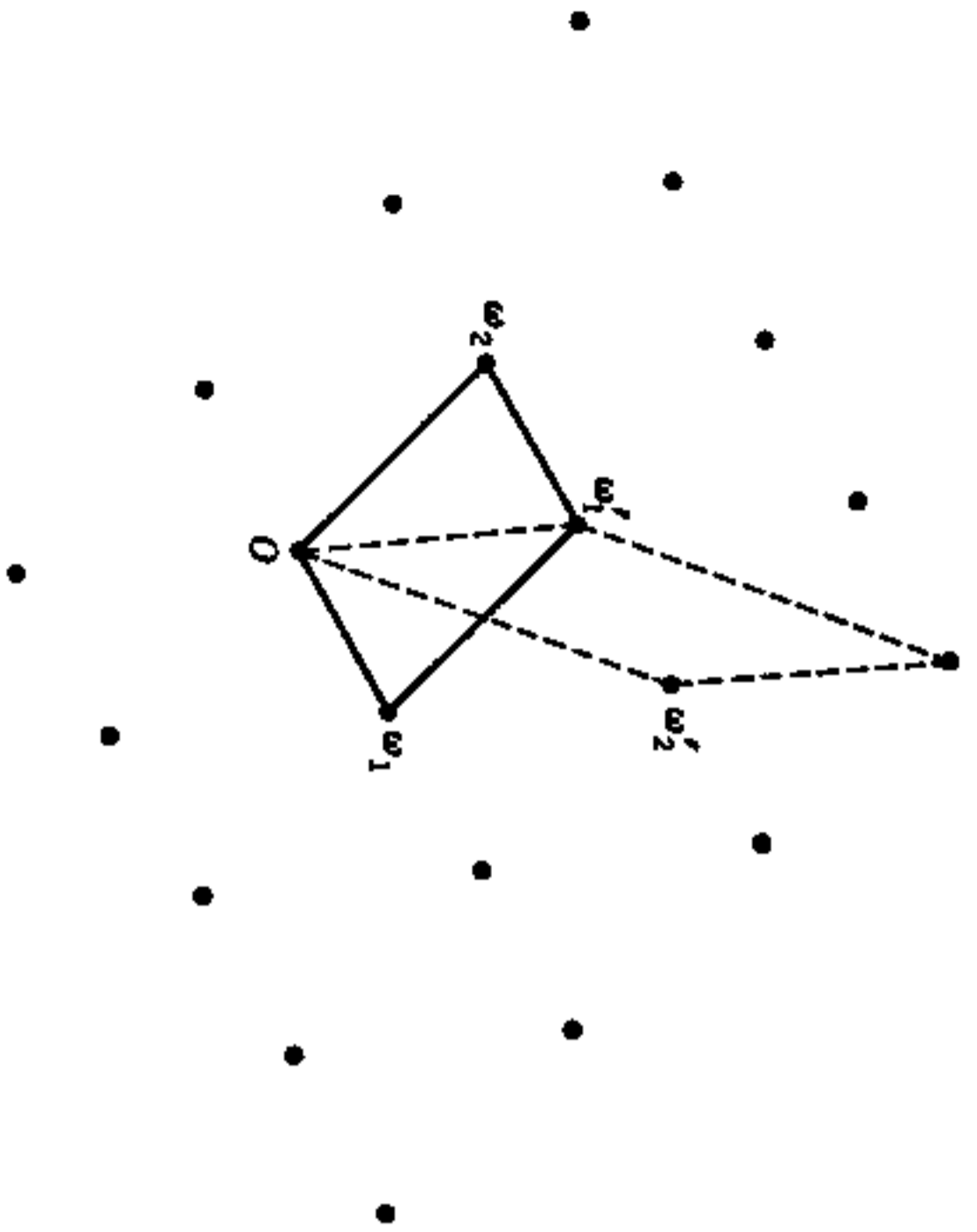
FIG. 7-1. Period module.
