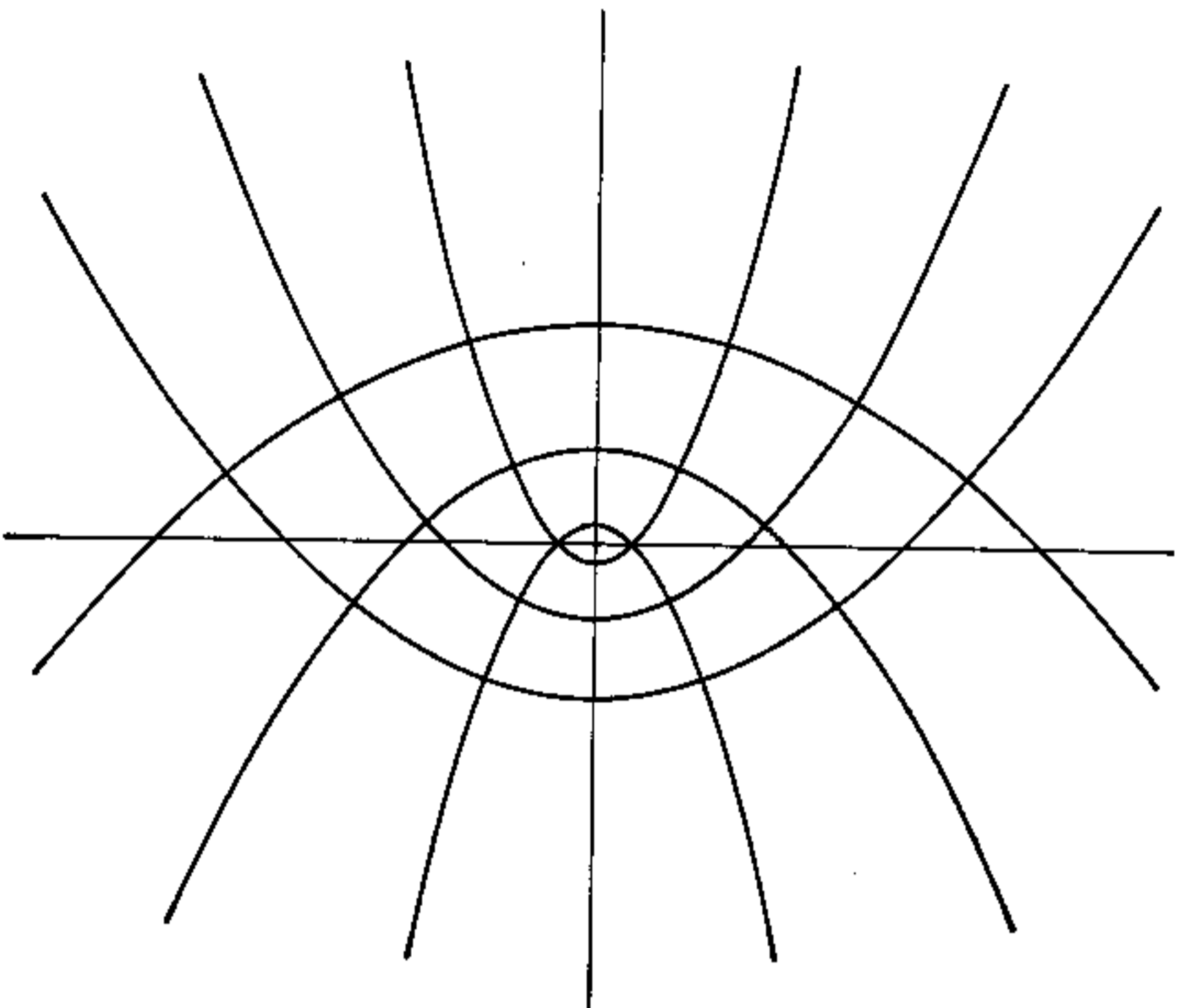
FIG. 1-6. w -plane.
