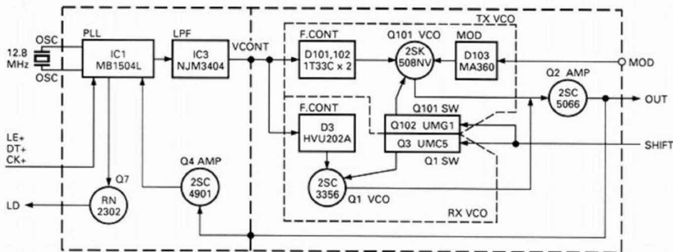
Fig. 10 Main PLL VCO block diagram (IC201 : L78-0363-08)
