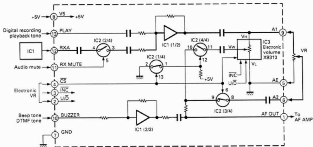
Fig. 13 RX audio circuit (IC2 : W02-1829-08)
