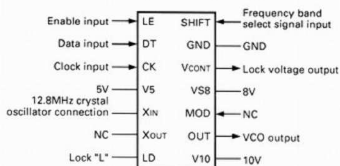
Fig. 9 Sub PLL VCO pin description (IC203 : L78-0351-08)
