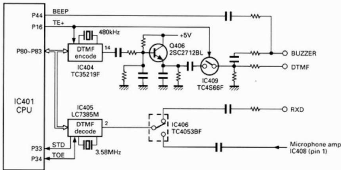
Fig. 23 DTMF input/output
