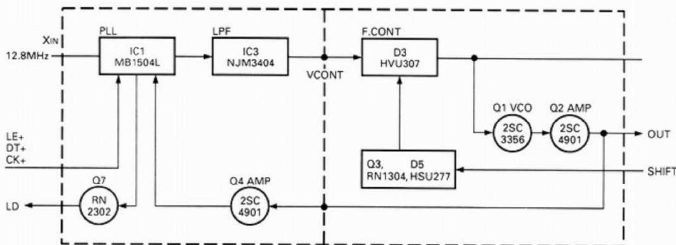
Fig. 11 Sub PLL VCO block diagram (IC203 : L78-0351-08)
