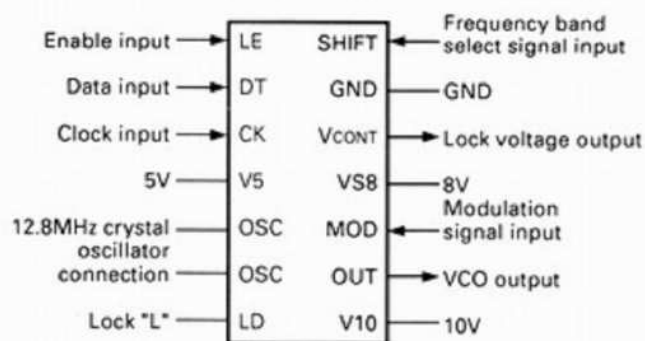
Fig. 8 Main PLL VCO pin description (IC201 : L78-0363-08)
