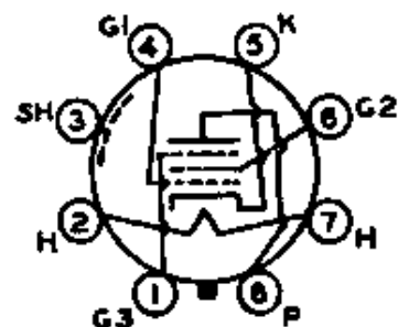
6AG7
