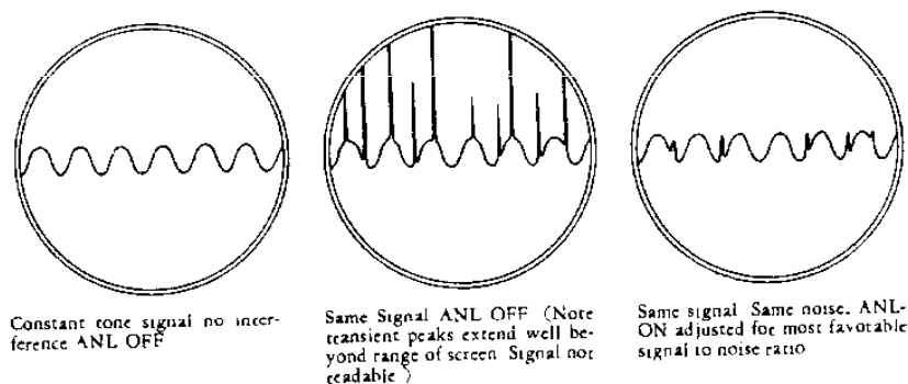
FIG. 6—NOISE LIMITER ACTION
