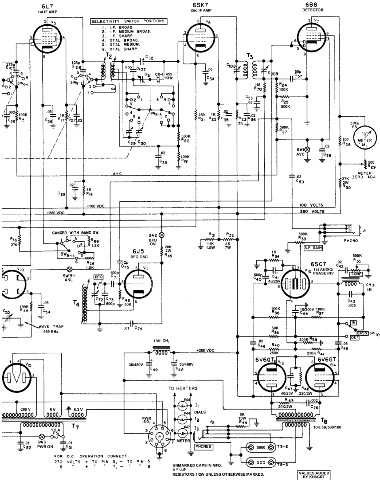
FIG. 13—SX28—SCHEMATIC
