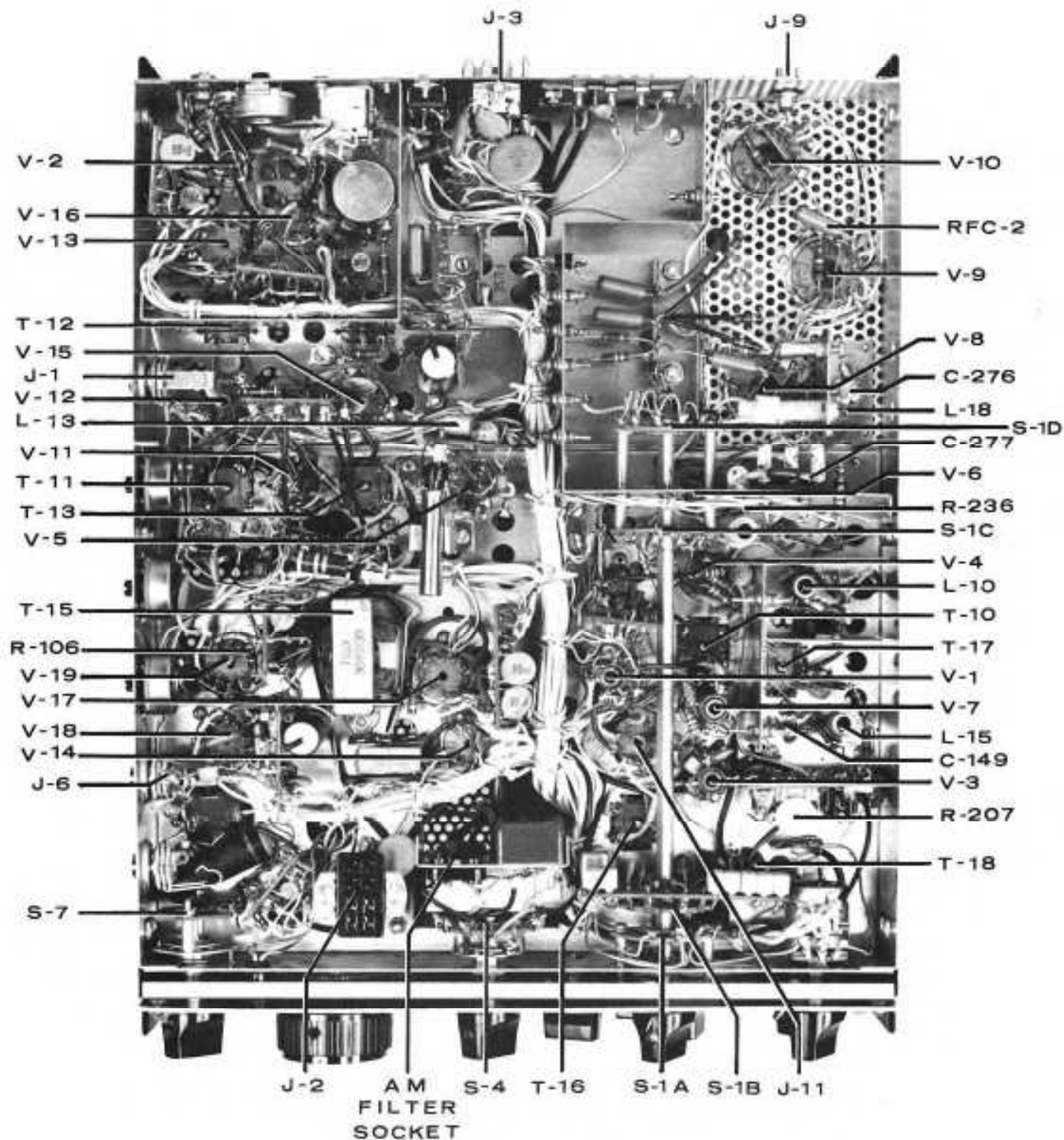
FIG.13- BOTTOM VIEW
