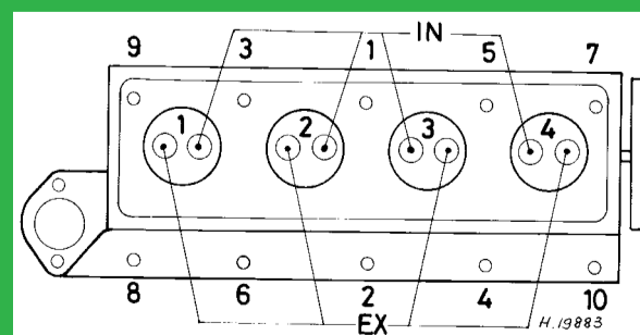
1297 cm 3 , OHV
