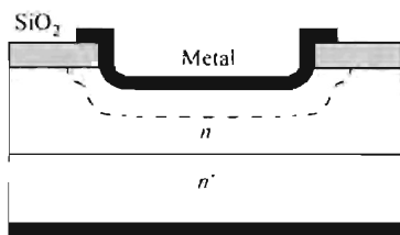
(d) Moat-etched
