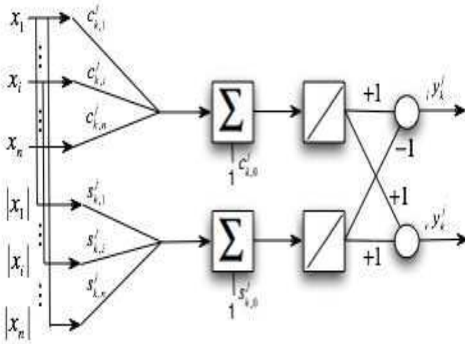
Fig. 1. Interval Type-1 Fuzzy Neuron (IT1FN)
