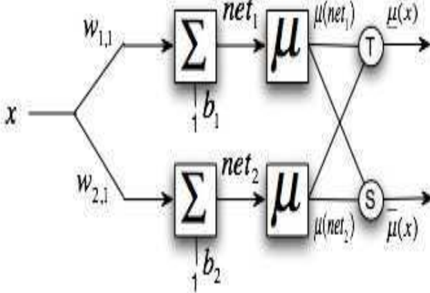
Fig. 2. Interval Type-2 Fuzzy Neuron (IT2FN)
