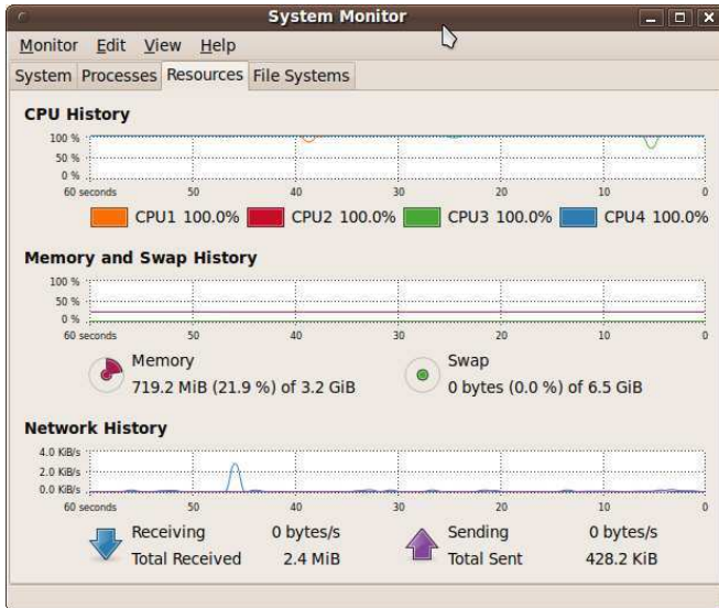
Fig. 14. CPU usage
